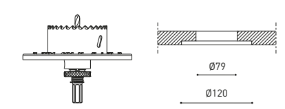
TRIMLESS TOOL D79 X D120mm A478-00-05
