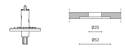
TRIMLESS TOOL D20 X D52mm A478-00-01
