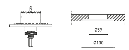
TRIMLESS TOOL D59 X D100mm A478-00-03
