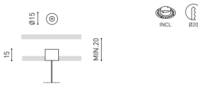
TRIMLESS TOOL D20 X D52mm A478-00-01
