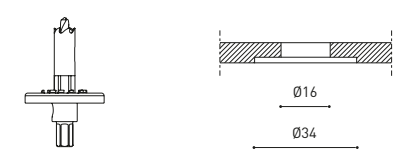
TRIMLESS TOOL D16 X D34mm A478-00-00
